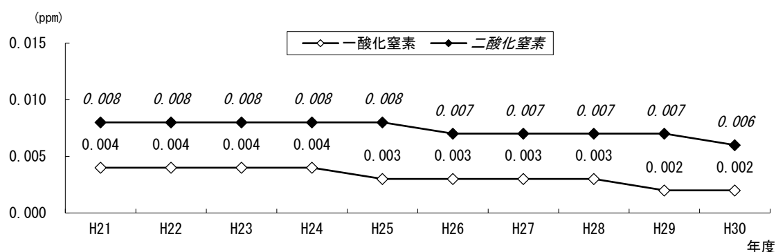
■一酸化窒素及び二酸化窒素濃度の年平均値の経年変化
