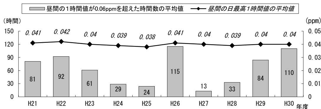
■道内の光化学オキシダント濃度の昼間の日最高1時間値の年平均値経年変化
